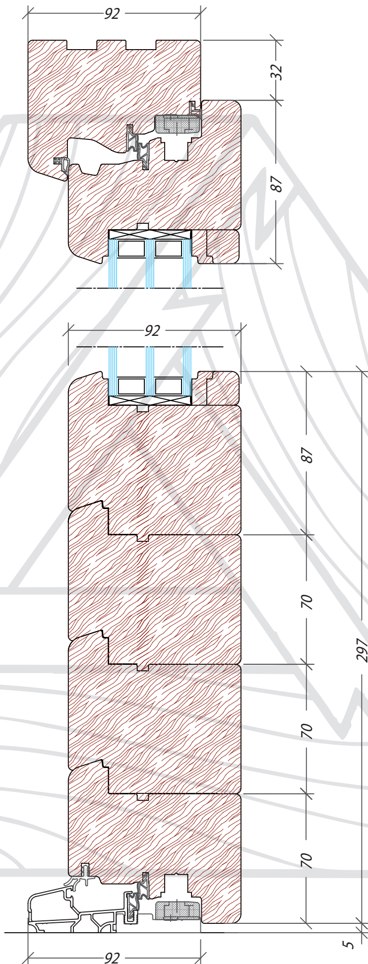
sezione verticale portafinestra
